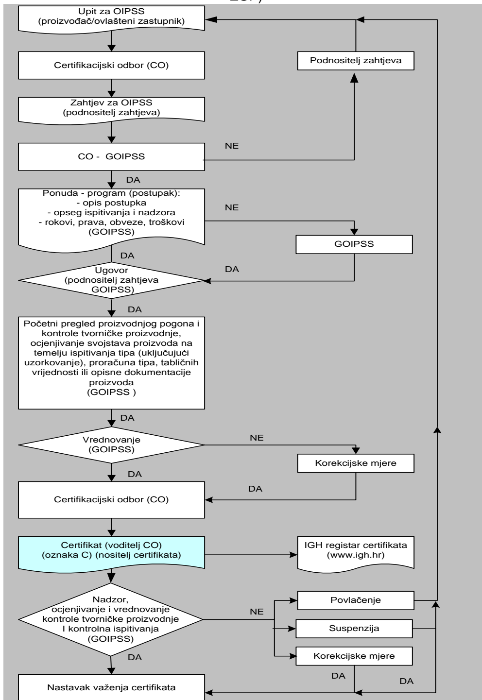
Dijagram toka - Procedura ocjenjivanja i provjere stalnosti svojstava i dodjele certifikata – (sustav 1+, ZGP)
